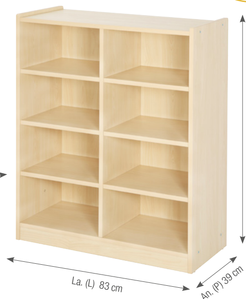
8 compartimentos – estantes fijos 8 scomparti – ripiani fissi
